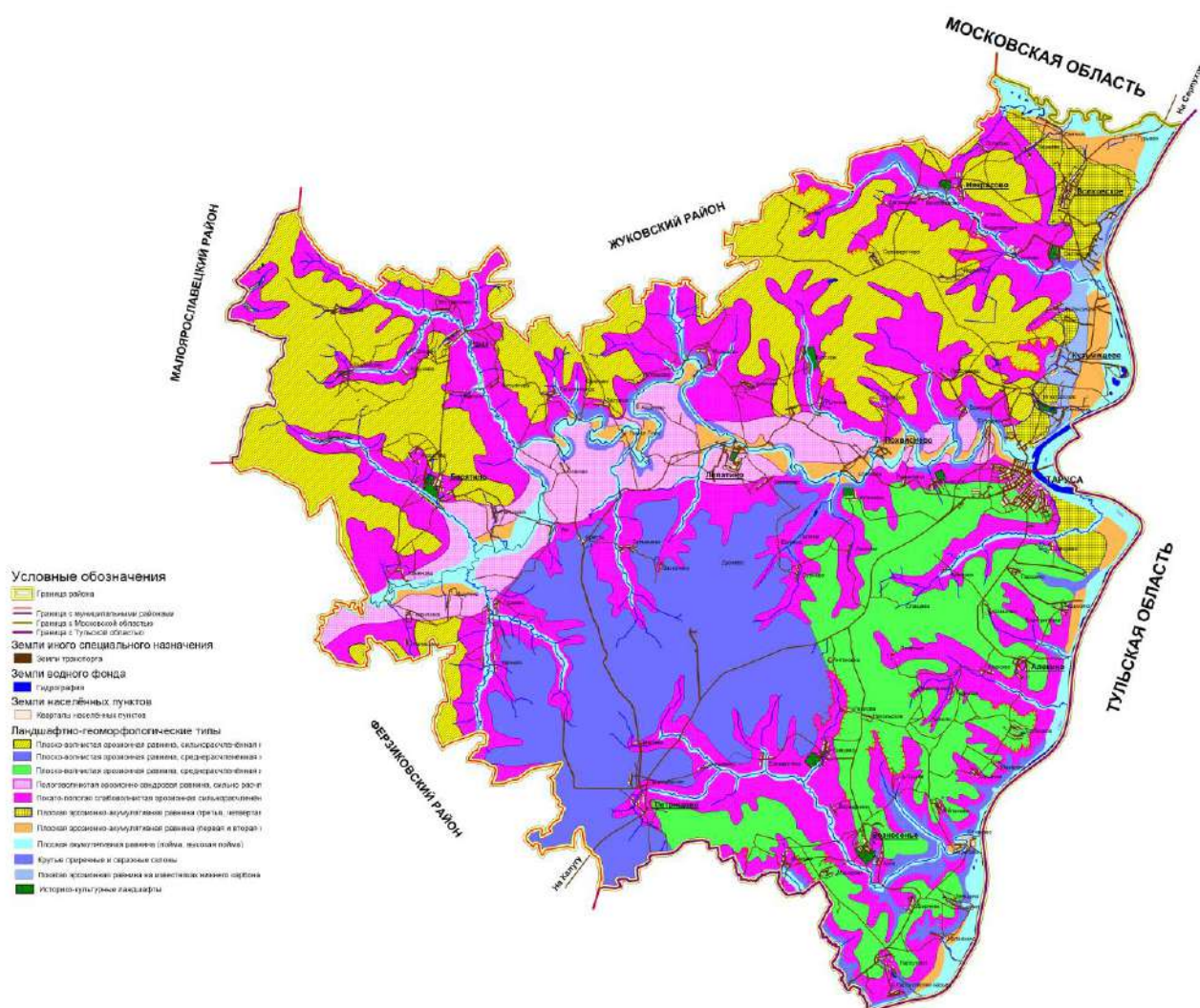
Ландшафтно-геоморфологическая карта М 1 : 50 000
